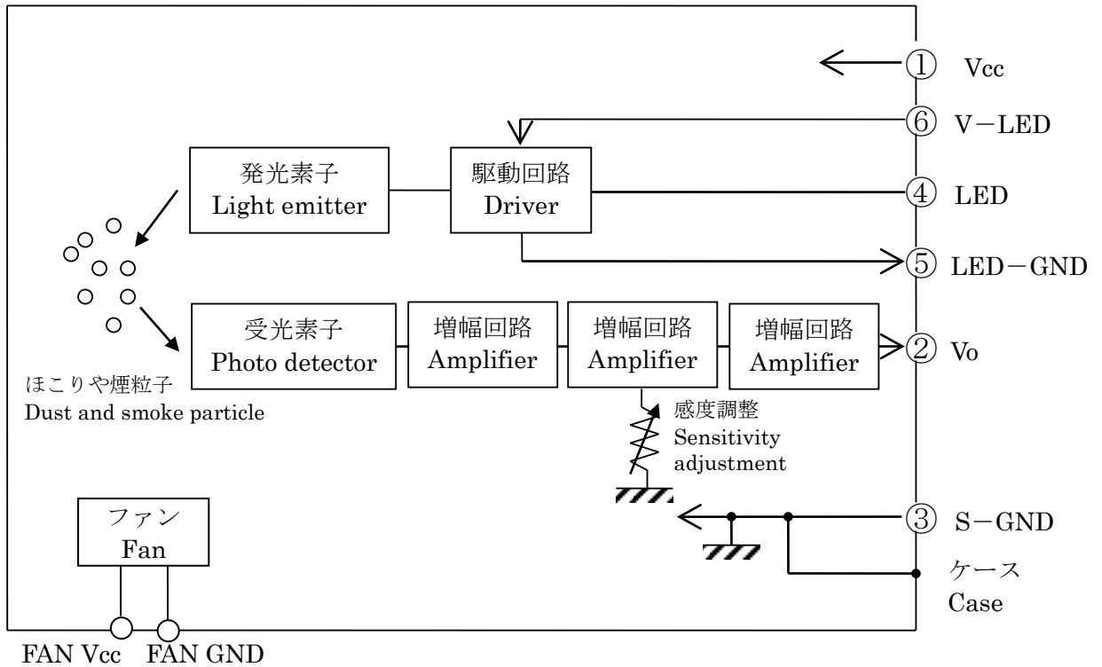
回路ブロック図 (Circuit block diagram)
